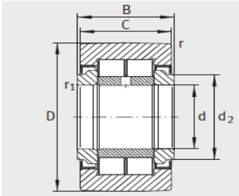
NNTR (优化的 INA 轮廓形状)
