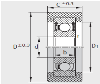
KLRZ..-2RSR KLRZ..-2Z
