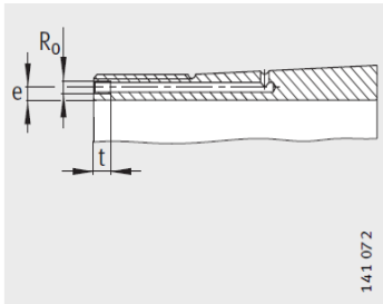
液压紧定套 安装尺寸
