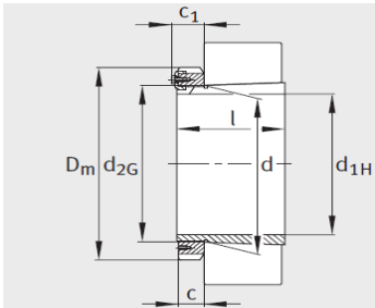
锥度为 1 : 12 (H240、 H241 系列, 锥度为 1 : 30)
