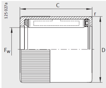
HF..-R、 HF..-KF-R 带滚花
